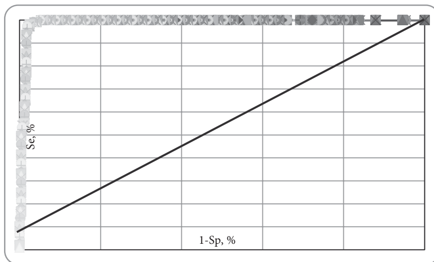
Рис. 6. ROC-кривая
